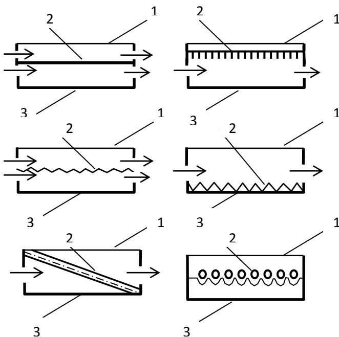
Рис. 4 Види плоских сонячних колекторів 1 – прозоре покриття; 2 – плита або трубка; 3 – корпус.
