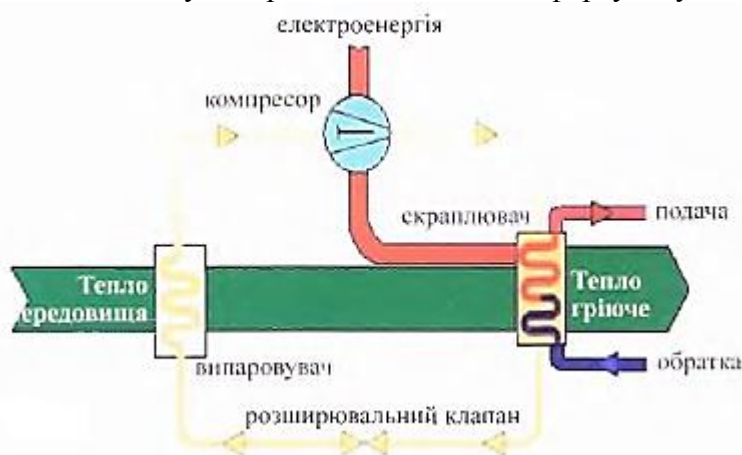
Рис. 3 – Принцип роботи теплового насоса
