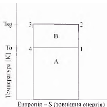
Рис.1 - Цикл Карно
