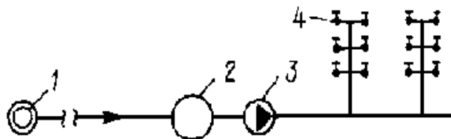
1 – геотермальна свердловина; 2 – бак акумулятор; 3 – мережний насос; 4 – водозабірний кран гарячої води.
