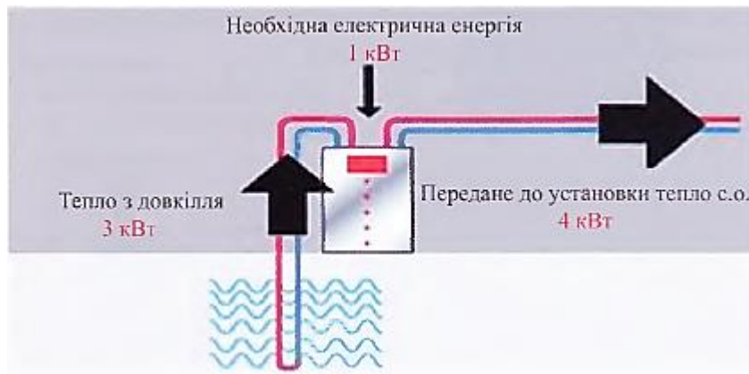
Рис. 2 - Схема розподілу енергії в теплонасосній установці
