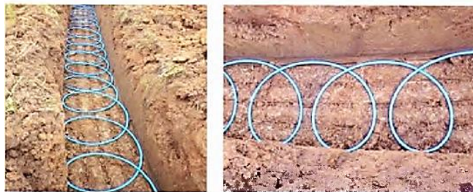
Рис. 4 Спосіб укладки горизонтального ґрунтового теплообмінника [19]
