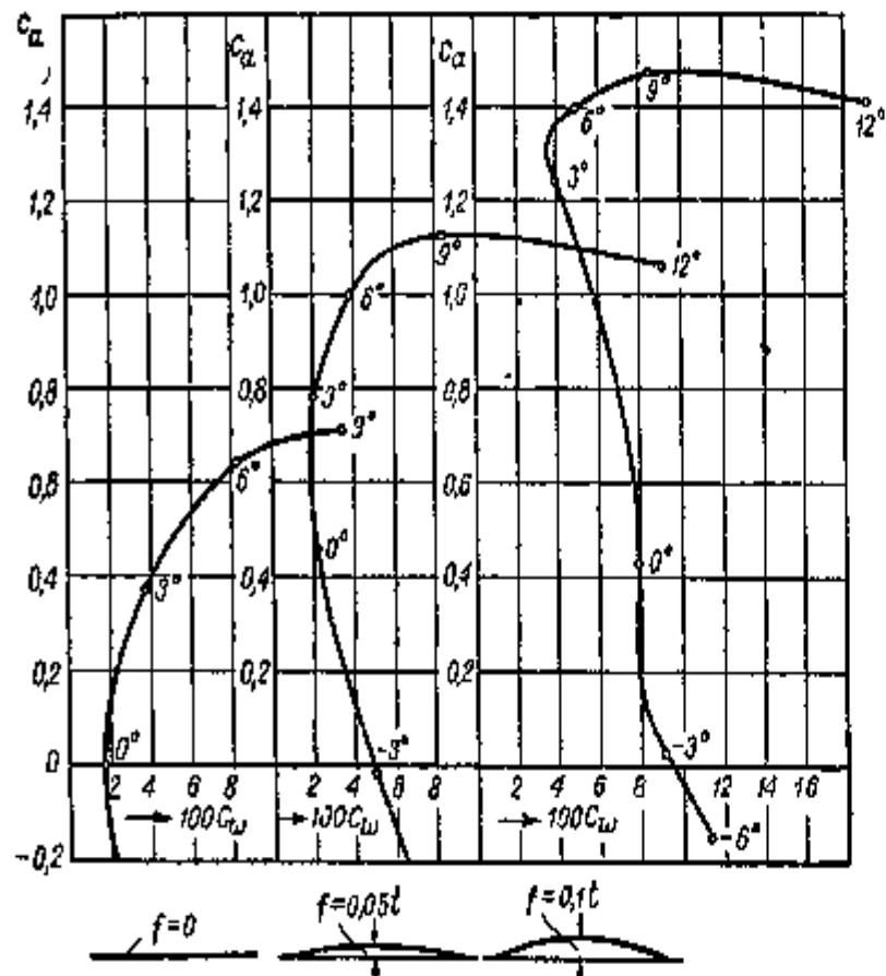
Рис. 2.4 Поляри Лілієнталя для лопатей нескінченної довжини.
