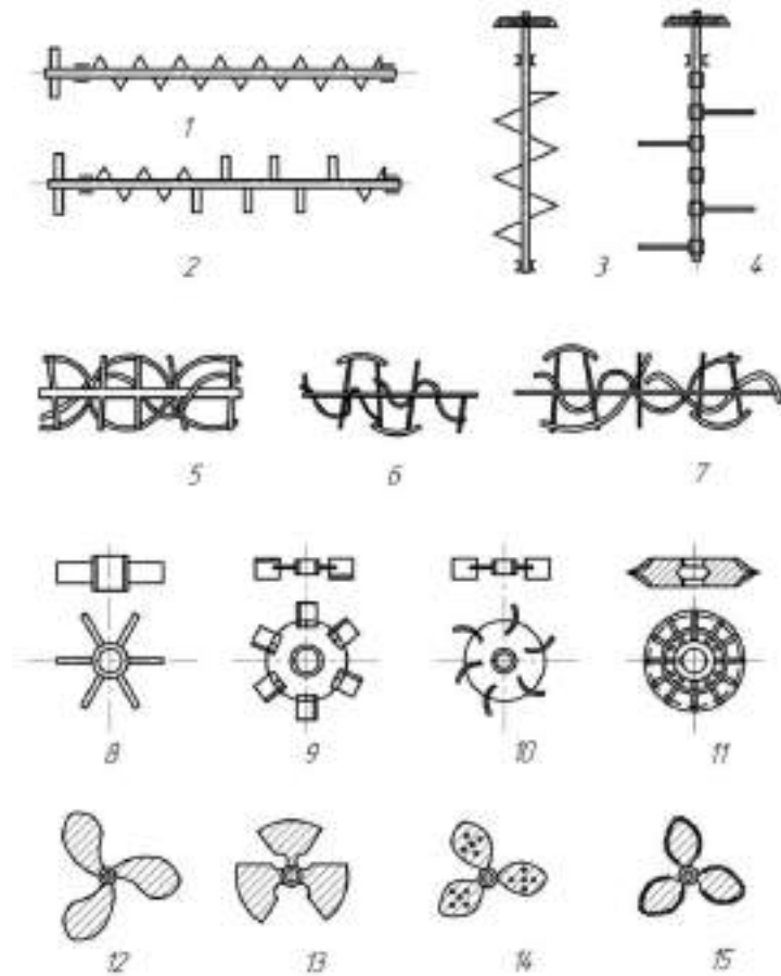
Рисунок 7.3. Типи робочих органів змішувачів: 1, 2, 3 – шнекові; 4 – лопатеві; 5, 6, 7 – стрічкові гвинтові; 8, 9, 10, 11 – турбінні; 12, 13, 14, 15 – пропелерні.
