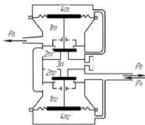
Рисунок 10.12. Схема вібропульсатора
