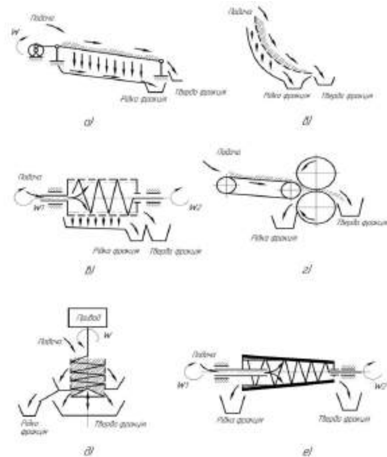
Рисунок 8.5. Схеми обладнання для обробки гною: а – віброгрохот; б – дугове сито; в – фільтруюча центрифуга; г – валкові зневоднювачі; д – шнековий прес; е – осаджувальна центрифуга
