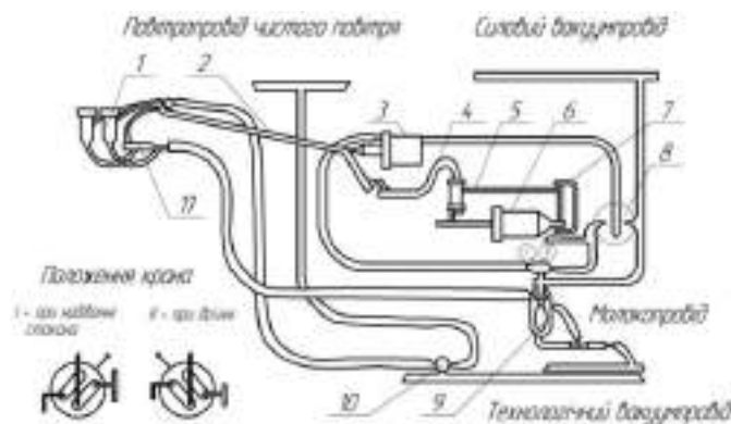
Рисунок 11.6. Маніпулятор доїння МД-Ф-1:
