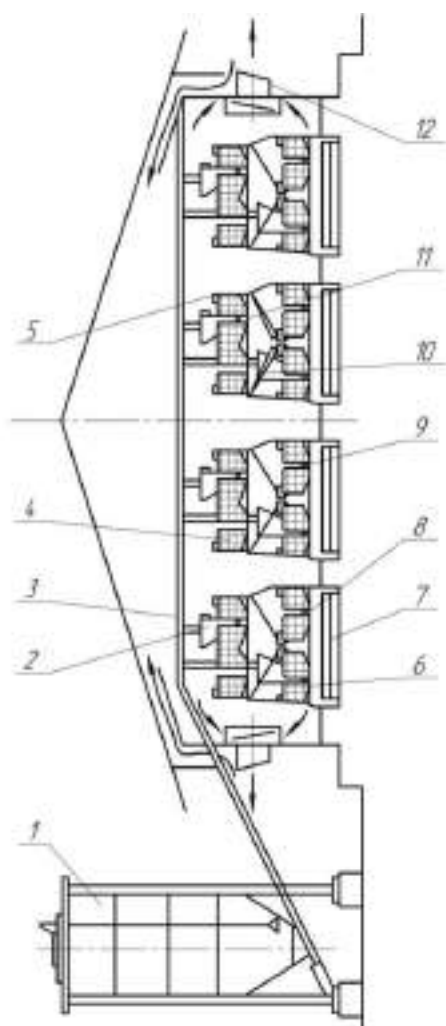
Рисунок 13.3. Поперечний перетин пташника з двоярусними клітковими батареями обладнання типу ККТ: 1 – зовнішній бункер для зберігання корму; 2 – бункер-дозатор кормороздавача; 3 – лінія завантаження кормів; 4 – верхній
