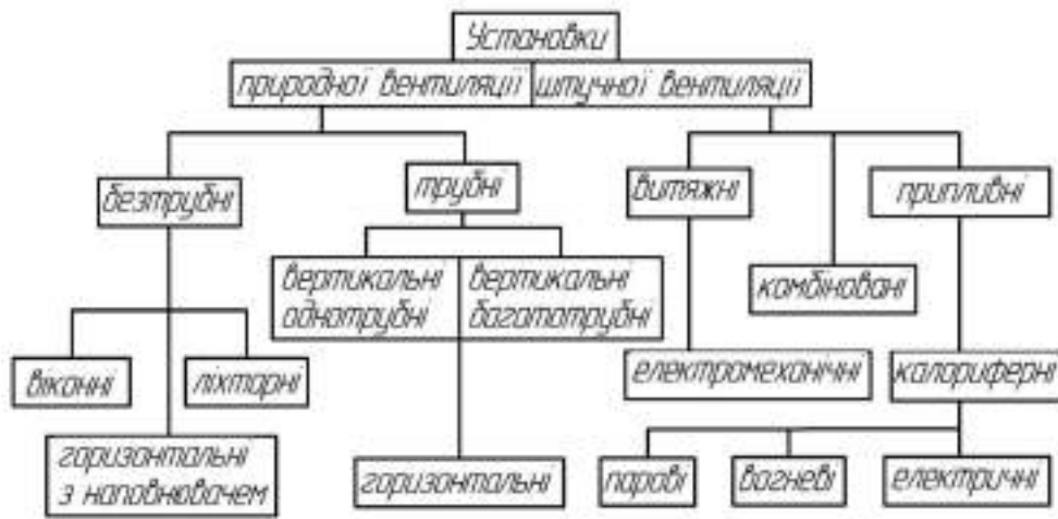
Рисунок 9.1. Класифікація вентиляційних установок
