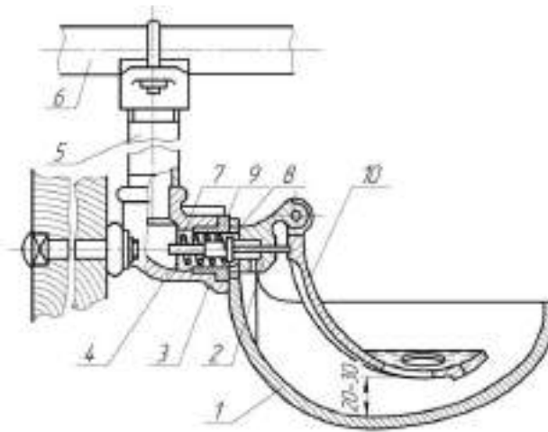
Рисунок 9.5. Автонапувалка ПА-1: 1 – напувальна чаша; 2 – клапанна коробка; 3 – корпус; 4 – решітка; 5 – стояк; 6 – труба; 7 – пружина; 8 – клапан; 9 – втулка; 10 – натискна педаль
