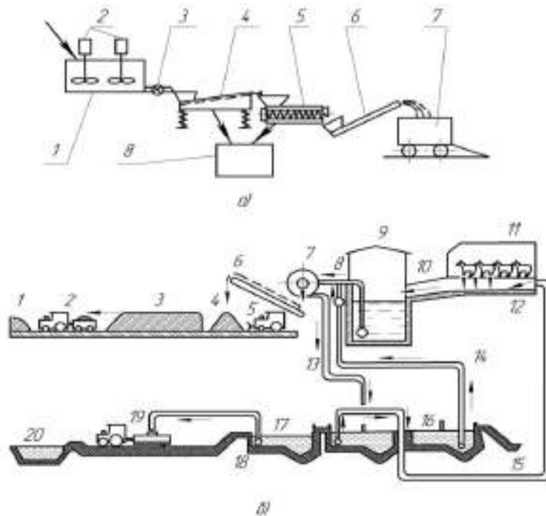
Рисунок 8.6. Схеми поточкових ліній переробки рідкого гною з поділом на фракції: а – лінія з віброгрохотом і шнековим фільтр-пресом: 1 – резервуар; 2 – лопатеві мішалки; 3 – заслінка; 4 – віброгрохот; 5 – шнековий прес-фільтр; 6 – скребковий транспортер; 7 – транспортний засіб; 8 – гноївкозбірник; б – лінія з фільтруючою центрифугою: 1 – штабель; 2 – причеп; 3,4 – бурти; 5 – бульдозер; 6 – стрічковий транспортер; 7 – транспортний засіб; 8 – гноєпровід; 9 – насосна станція; 10 – поперечний колектор; 11 – тваринницьке приміщення; 12 – гноєприймальний канал; 13 – трубопровід; 14 – зворотний трубопровід; 15 – змивний трубопровід; 16,17 – відстійники-накопичувачі; 18 – заглибний насос; 19 – цистерна; 20 – польовий гноєзбірник
