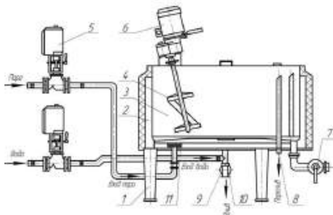
Рисунок 12.14. Схема ванни тривалої пастеризації: 1 – опора; 2 – корпус; 3 – ванна; 4 – мішалка; 5 – електромагнітний клапан; 6 – привод мішалки; 7 – кран; 8 – переливна труба; 9 – вентиль для зливання води; 10 – трубка; 11 – паророзподільна головка
