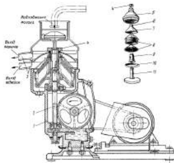
Рисунок 12.17. Загальний вигляд сепаратора ОСБ-1000 і деталі барабана: 1 – станина; 2 – вал вертикальний (веретено); 3 – канали; 4 – накидна гайка; 5 – гвинт регулювання жирності вершків; 6 – корпус; 7 – верхня тарілка; 8 – пакет роздільних тарілок; 9 – тарілотримач; 10 – гумове кільце; 11 – основа барабана з центральною трубою
