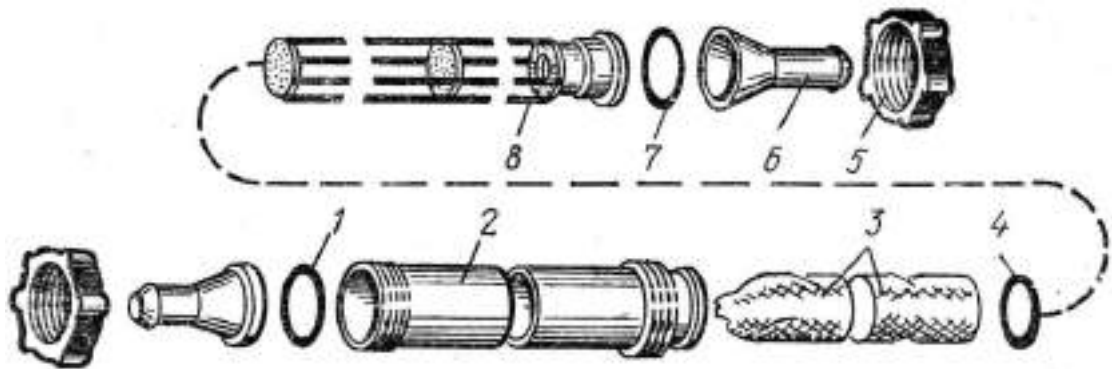
Рисунок 12.2. Циліндричний фільтр для очищення молока: 1, 7 – ущільнювальні прокладки; 2 – корпус; 3 – фільтруючий елемент; 4 – кільце; 5 – гайка; 6 – перехідник; 8 – каркас
