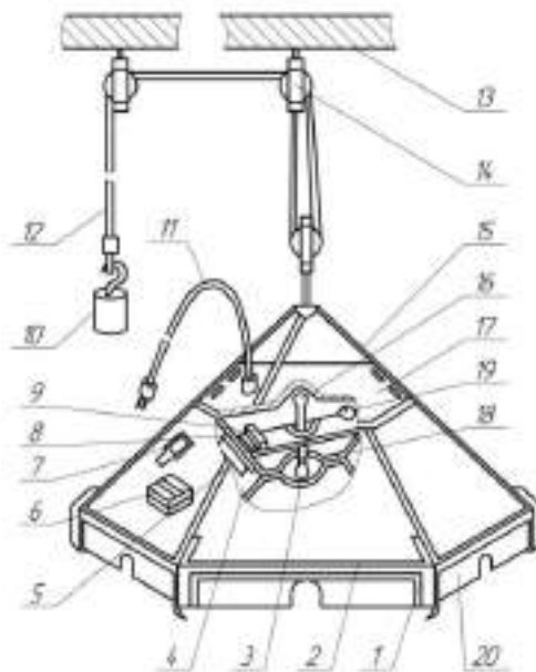
Рисунок 13.5. Брудер БП-1
