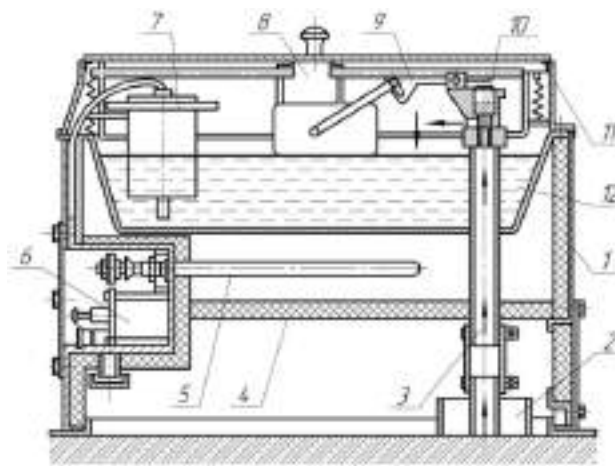
Рисунок 21.5. Автонапувалка групова АГК-4А з електропідігрівом: 1 – корпус; 2 – утеплювальна труба; 3 – водовідвідна труба; 4 – ізоляція; 5 – нагрівник; 6 – блок заземлення; 7 – терморегулятор; 8 – поперечка; 9 – поплавковий механізм; 10 – клапан; 11 – кришка; 12 – напувальна чаша
