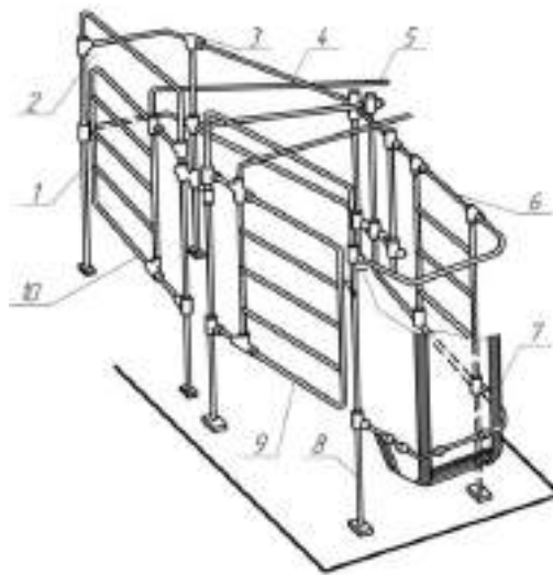
Рисунок 11.4. Станок доїльної установки УДТ-6 типу «Тандем» (правий): 1 – стояк; 2 – щиток; 3 – косинець; 4, 6 – труби; 5 – тяга дверей; 7 – годівниця; 8 – стояк вертикальний; 9 – двері випускні; 10 – двері впускні
