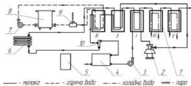
Рисунок 12.15. Схема пастеризаційно-охолоджувальної установки:
