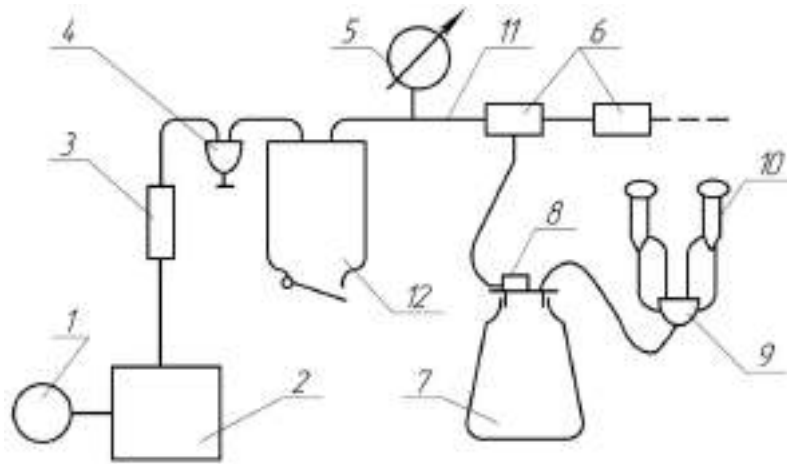
Рисунок.10.1. Схема доїльної машини:
