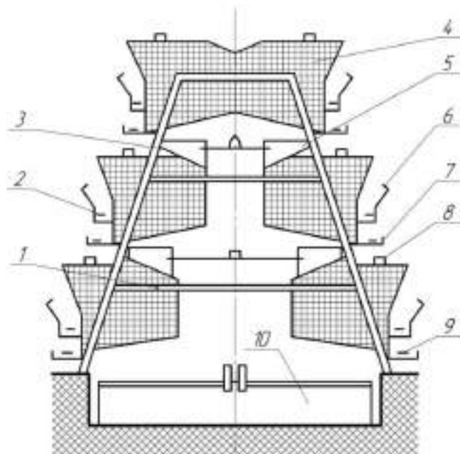
Рисунок 13.4. Поперечний перетин кліткової батареї БКН-3:
