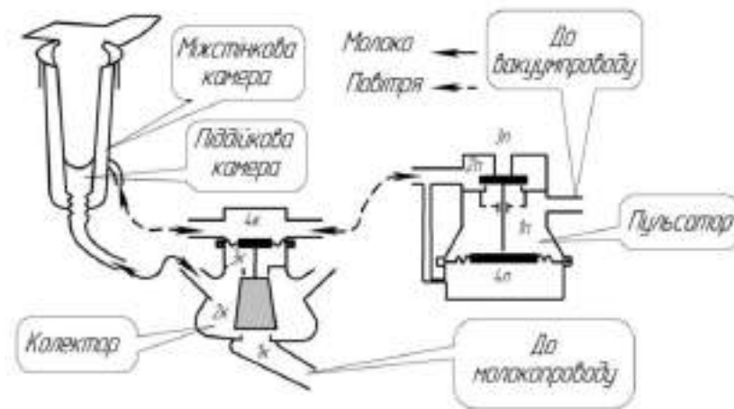
Рисунок 10.3. Схема роботи доїльного апарата
