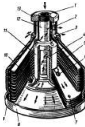
Рисунок 12.16. Схема розподілення молока в барабані сепаратора: 1 – вхідний отвір центральної трубки; 2 – отвір для виходу вершків; 3 – отвір для виходу відвійок; 4 – бічний канал; 5 – верхня роздільна тарілка; 6 – вертикальні канали; 7 – тарілки; 8 – корпус; 9 – кришка; 10 – отвір; 11 – тарілкотримач; 12 – трубка; 13 – гайка
