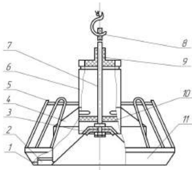
Рисунок 13.6. Бункерна годівниця ЦБК-2-06А:
