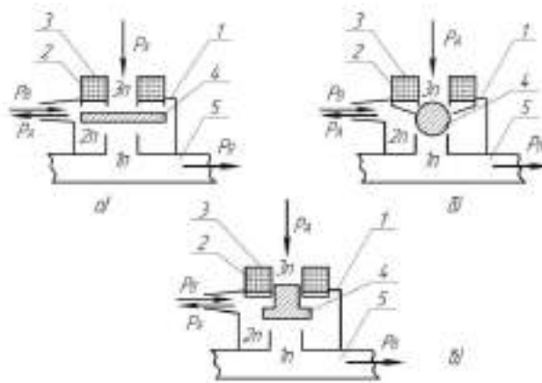
Рисунок 10.9. Схеми електромагнітних пульсаторів:
