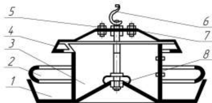
Рисунок 13.7. Годівниця для мінерального підкорму і гравію КЦБ-2А: 1 – піддон; 2 – кільце; 3 – бункер; 4 – козирок; 5 – вісь; 6 – гак; 7 – кронштейн; 8 – різьбове з'єднання
