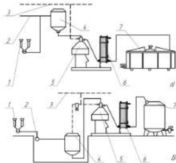
Рисунок 12.4. Схеми ліній очищення й охолодження молока для доїльних установок з верхнім (а) і нижнім (б) розташуванням молокопроводу: 1 – доїльний апарат; 2 – молокопровід; 3 – вакуум-провід; 4 – молокозбірник; 5 – відцентровий молокоочисник; 6 – пластинчастий охолоджувач; 7 – резервуар для молока
