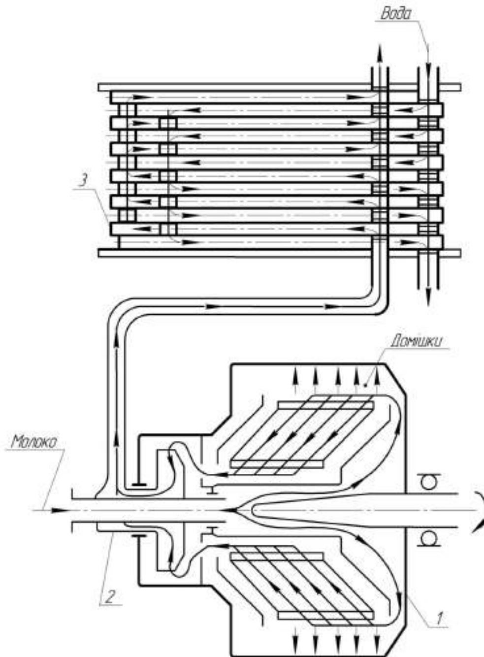
Рисунок 12.5. Технологічна схема очисника-охолоджувача ОМ-1А: 1 – відцентровий очисник; 2 – приймально-вивідний пристрій; 3 – пластинчастий охолоджувач
