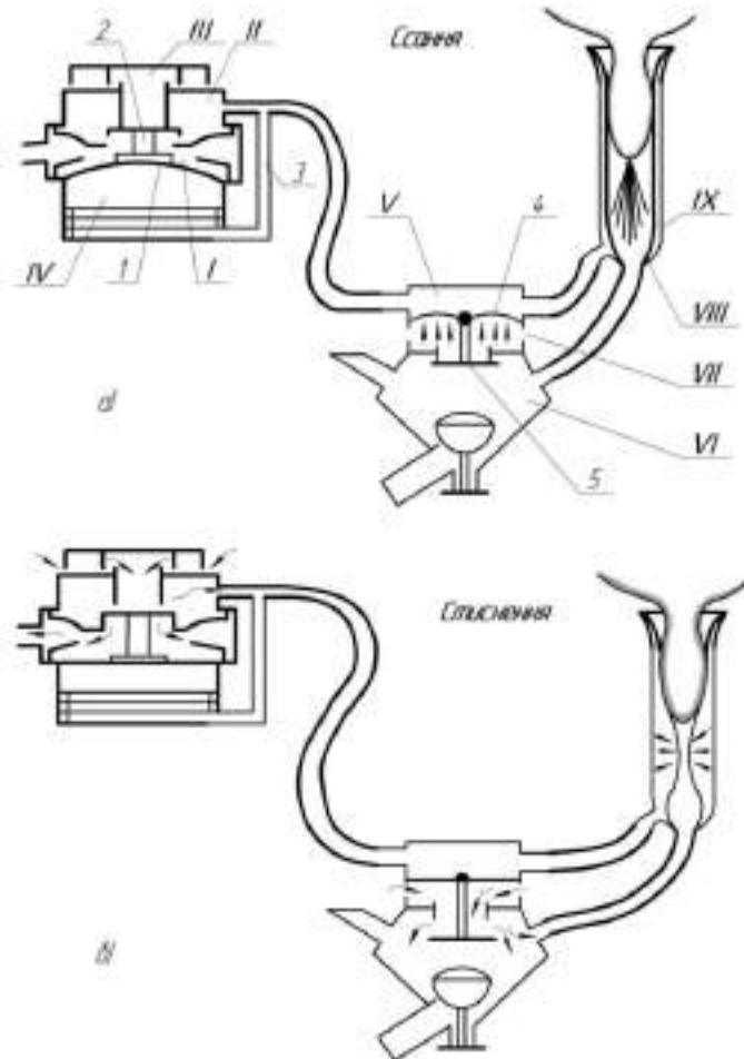
Рисунок 10.7. Схема роботи низьковакуумного доїльного апарата:
