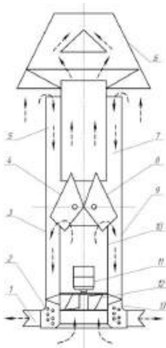
Рисунок 9.2. Схема припливно-витяжної установки: 1 – шарнірний відбивач; 2, 13 – нагрівальні елементи; 3 – циліндричний кожух; 4, 8 – заслінки поворотні напівциліндричні; 5, 7, – кільцеві припливні канали; 6 – козирок-відбивач; 10 – циліндр внутрішній; 11 – електродвигун; 12 – крильчатка вентилятора
