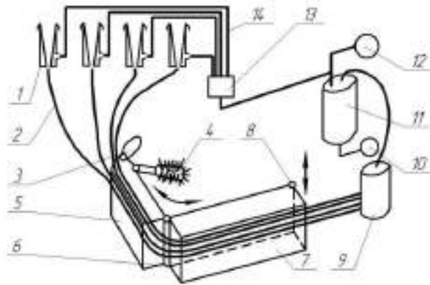
Рисунок 11.7. Принципова схема доїльного робота:
