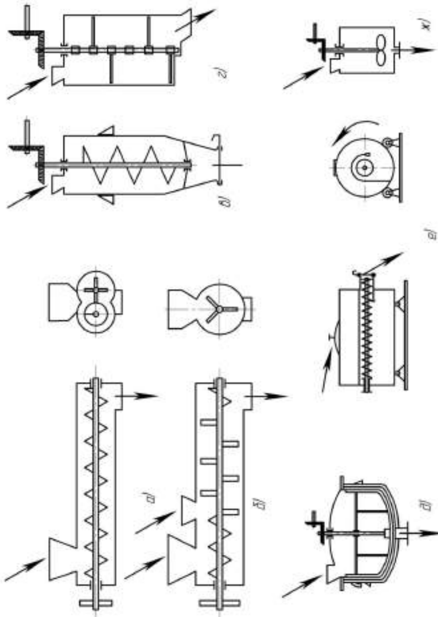
Рисунок 7.2. Схеми змішувачів кормів: а – шнековий горизонтальний неперервної дії; б – шнеково-лопатевий горизонтальний неперервної дії; в – шнековий вертикальний періодичної дії; г, д – лопатеві періодичної дії; е – барабанний періодичної дії; ж – пропелерний періодичної дії.
