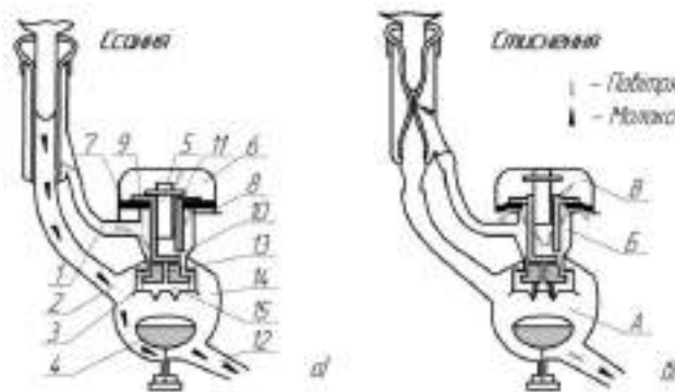
Рисунок 10.13. Схема роботи пульсоколектора:
