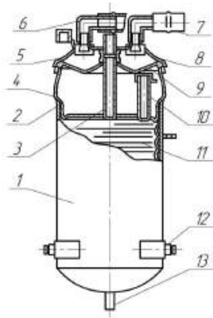
Рисунок 12.7. Вакуумний зрошувальний охолоджувач: 1 – корпус; 2, 5 – прокладки; 3 – патрубок під’єднання до вакуумної магістралі; 4 – молокоприймач; 6, 7 – патрубки підведення молока; 8 – кришка; 9 – фільтр; 10 – патрубок переливання молока; 11 – гофрована теплообмінна пластина; 12 – підвіска; 13 – патрубок відведення охолодженого молока
