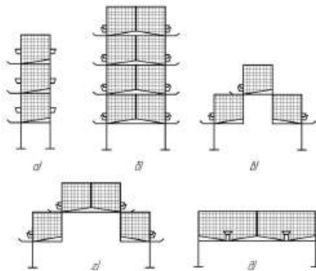
Рисунок 13.2. Схеми кліткових батарей:
