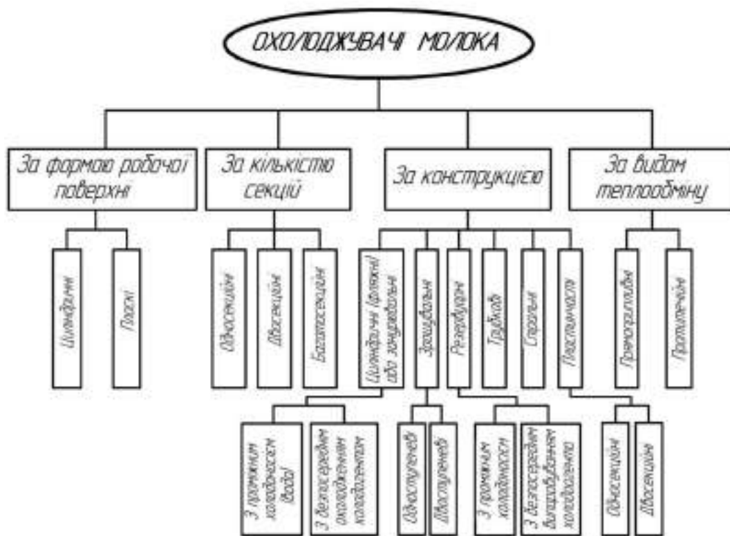
Рисунок 12.6. Класифікація обладнання для охолодження молока
