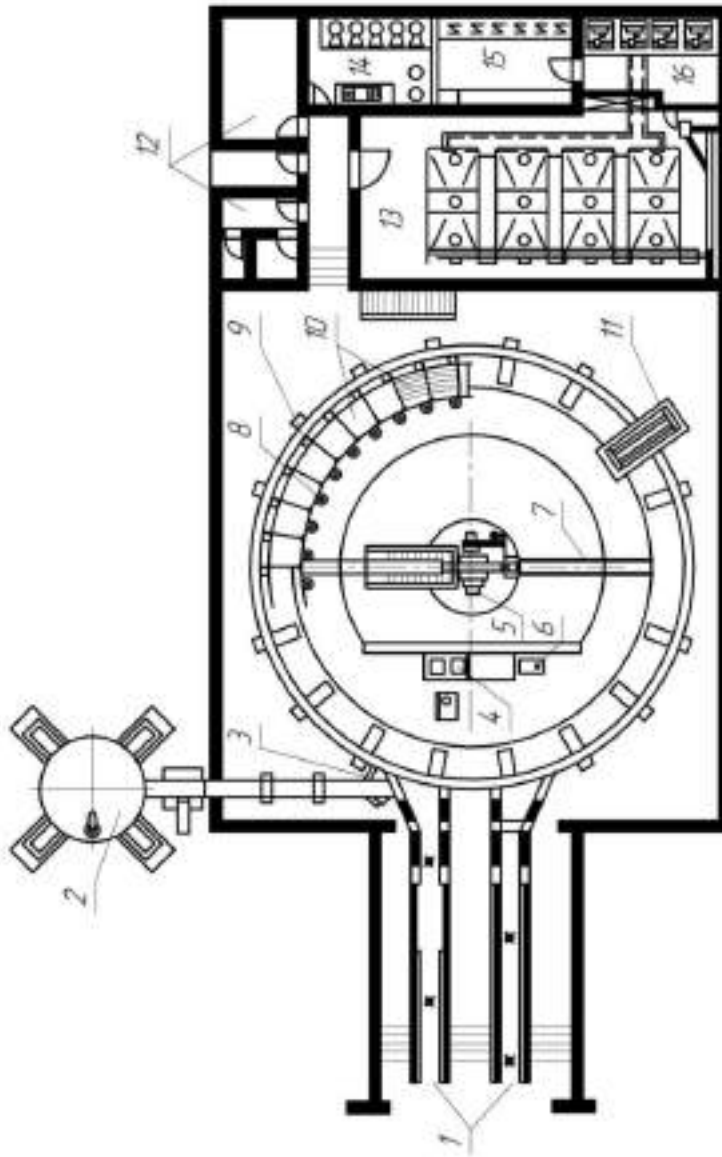
Рисунок 11.5. План-схема доїльної установки типу «Карусель»:
