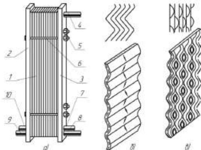
Рисунок 12.10. Пластинчастий теплообмінник (а) і схема руху потоку рідини в каналі, утвореному пластинами стрічково-потокowego (б) і сітчасто-потокowego (в) типів: 1 – комплект теплообмінних пластин; 2, 3 – плити; 4 – штанга; 5 – гайка; 6 – шпилька; 7, 10 – патрубки для підведення й відведення молока; 8, 9 – патрубки для підведення й відведення холодоносія
