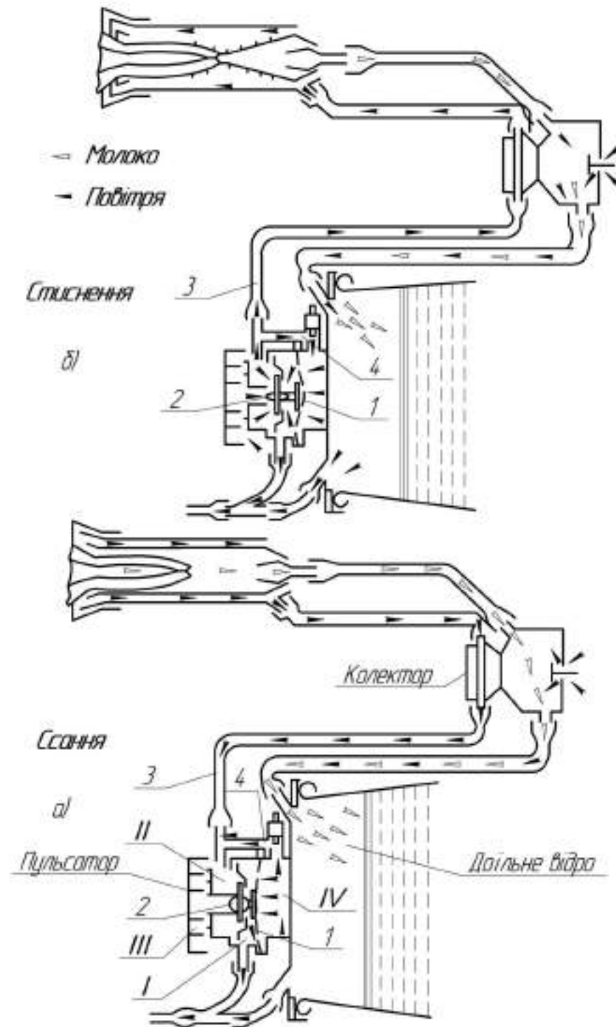
Рисунок 10.6. Схема роботи двотактного доїльного апарата:
