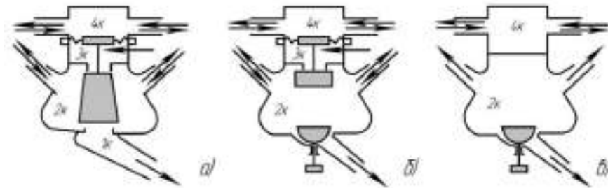
Рисунок 10.14. Схеми колекторів доїльних апаратів:
