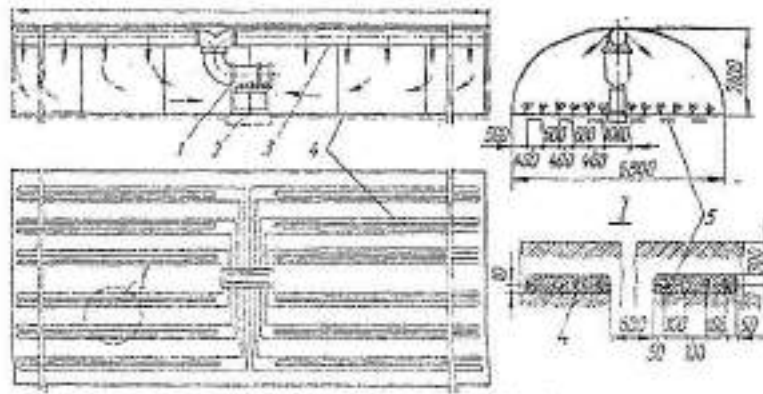
Рисунок 9 – Теплиця з ґрунтово-повітряним обігріванням: 1 – електрокалорифер; 2 – шафа керування; 3 – розподільний повітропровод; 4 – нагрівні проводи; 5 – цементно-піщаний розчин.
