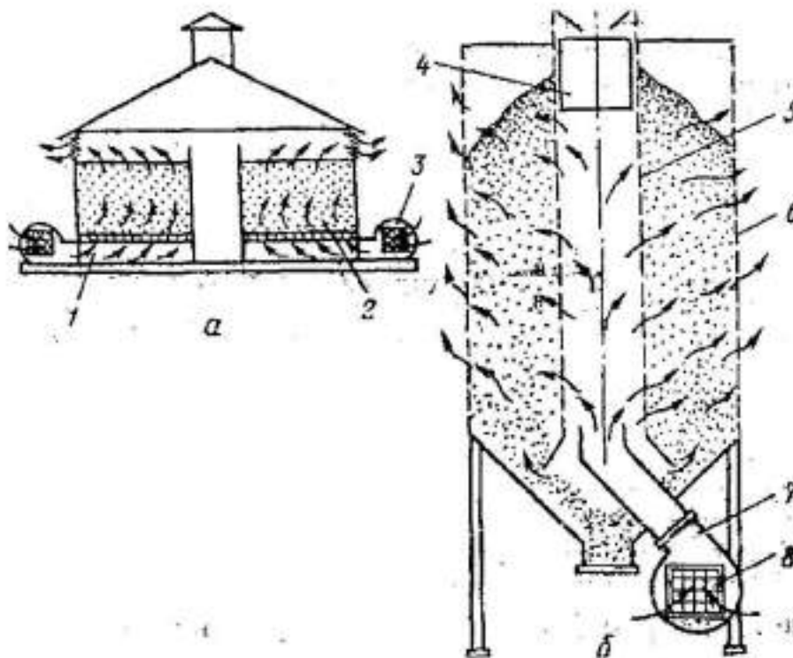
Рисунок 10 – Схеми активного вентилявання зерна в засіках (а) і бункерах активного вентилявання (б): 1 – повіторозподільний канал; 2 – засік із зерном; 3 – агрегат ВПЭ-6А; 4 – поршень-заглушка; 5 і 6 – внутрішній і зовнішній перфоровані циліндри; 7 – вентилятор; 8 – електрокалорифер.
