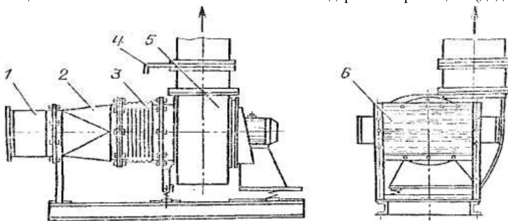
Рисунок 4 – Електрокалориферний агрегат серії СФОЦ:
