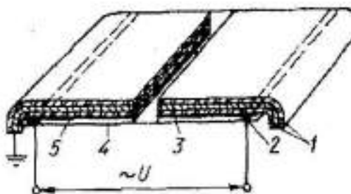
Рисунок 7 – Плівковий нагрівник:
