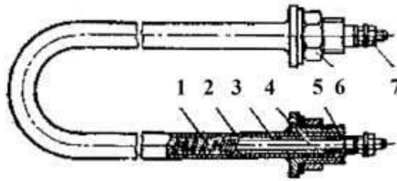
Рисунок 3 – Схематичне зображення трубчатого нагрівника (ТЕН):
