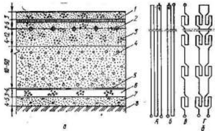
Рисунок 5 – Підлога з електрообігріванням:
