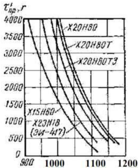
Рисунок 1 – Графік залежності строку служби дротового нагрівника від його розрахункової температури
