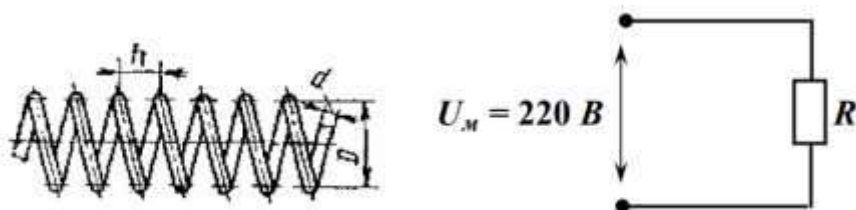
Рисунок 2 – Відкритий спіральний електронагрівник та сема його під'єднання
