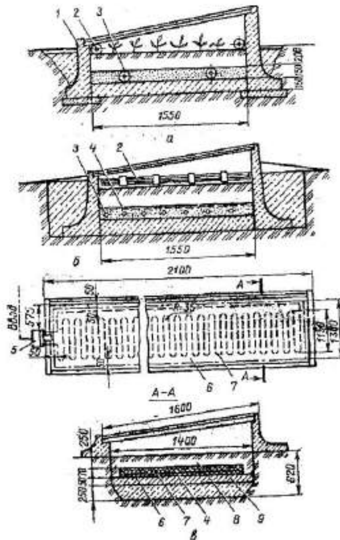
Рисунок 8 – Будова електрообігріву ґрунту і повітря в парниках:
