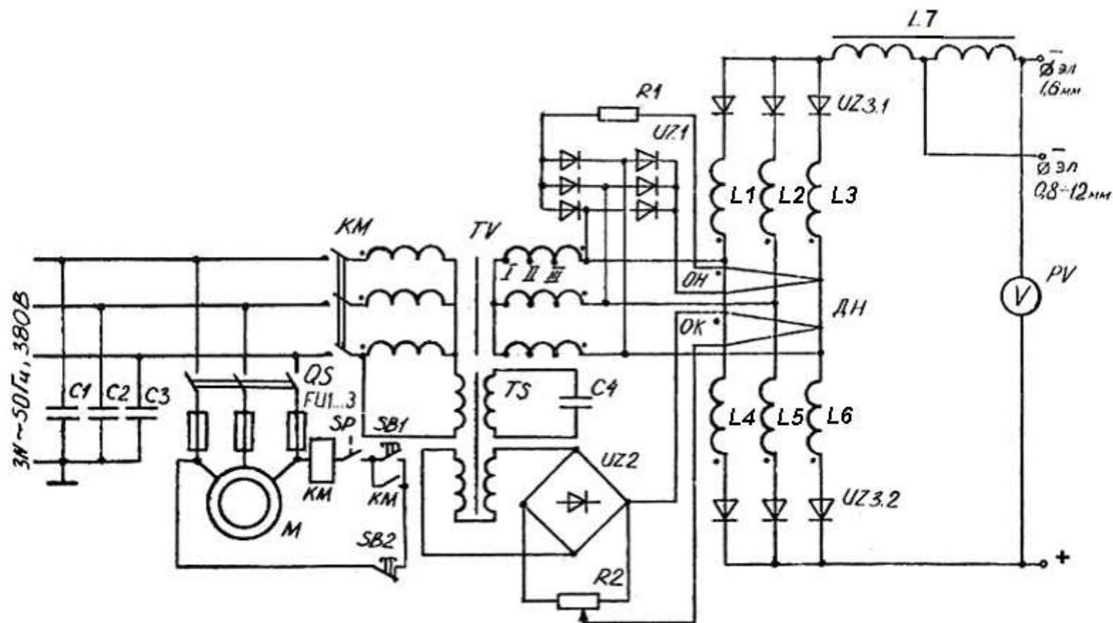
Рис8.1.Схема зварювального випрямляча ВДГ-301
