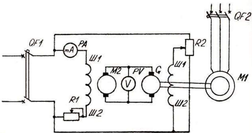
Рис1.2.Схемавмиканнядвигунавентилятора
