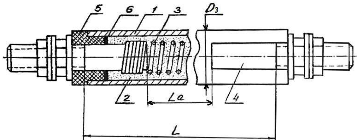
Рис.2.1. Розріз ТЕНа
