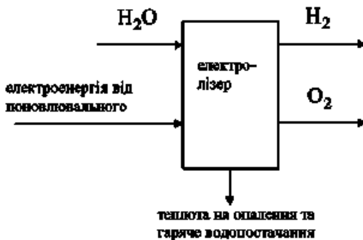
Рисунок 1 - Акумуляція енергії ПДЕ на основі водню
