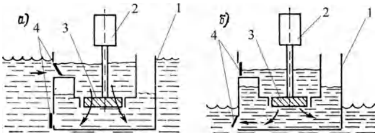
Рис. 3 - Випрямляч Расела:
