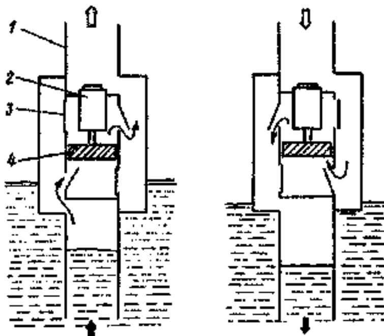
Рис.4 - Пневмобуй Масуді:
