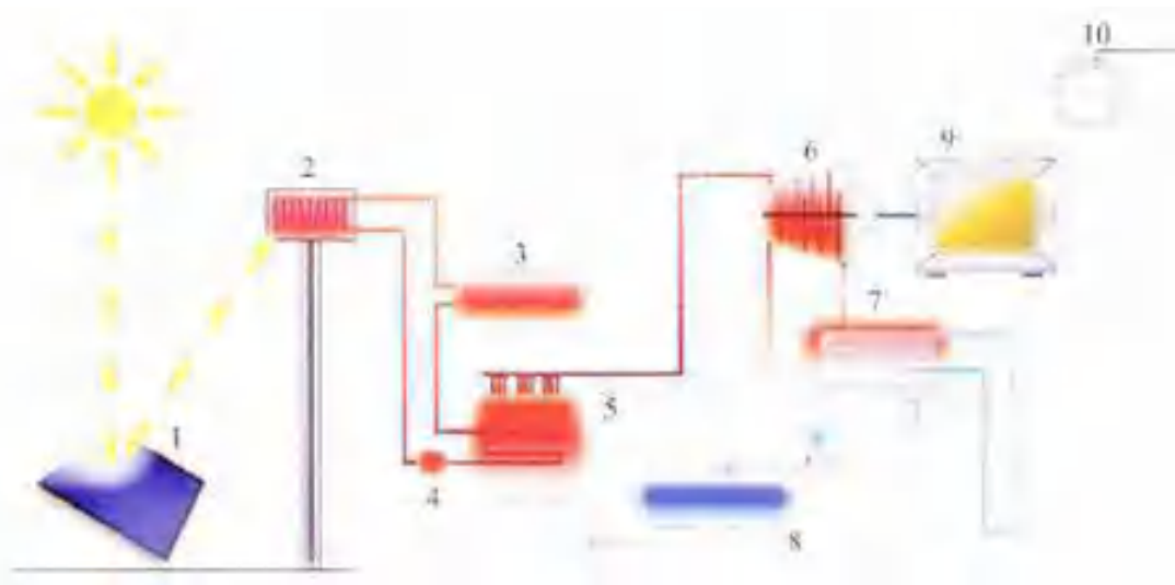
Рис. 1.4. Схема сонячної електростанції
