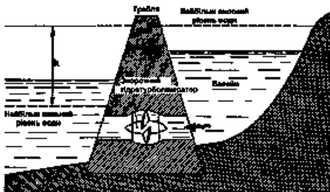
Рис. 9 - Спрощена схема ПЕС
