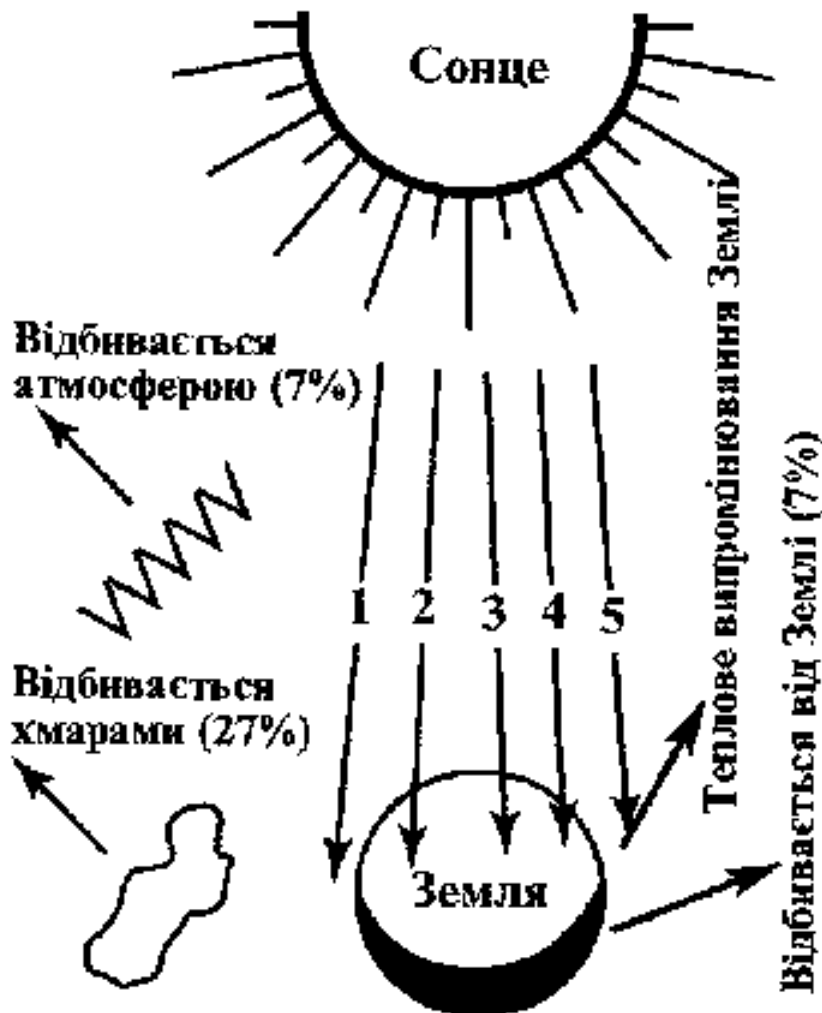
Рисунок 10.1 — Розподіл променевої енергії Сонця:
