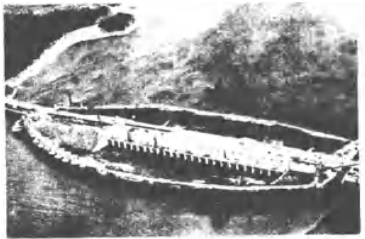
Рис. 11 - Припливна електростанція на річці Ранс
