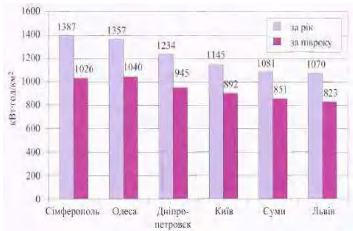
Рис. 1.3. Сумарна сонячна радіація на горизонтальну поверхню у різних містах України
