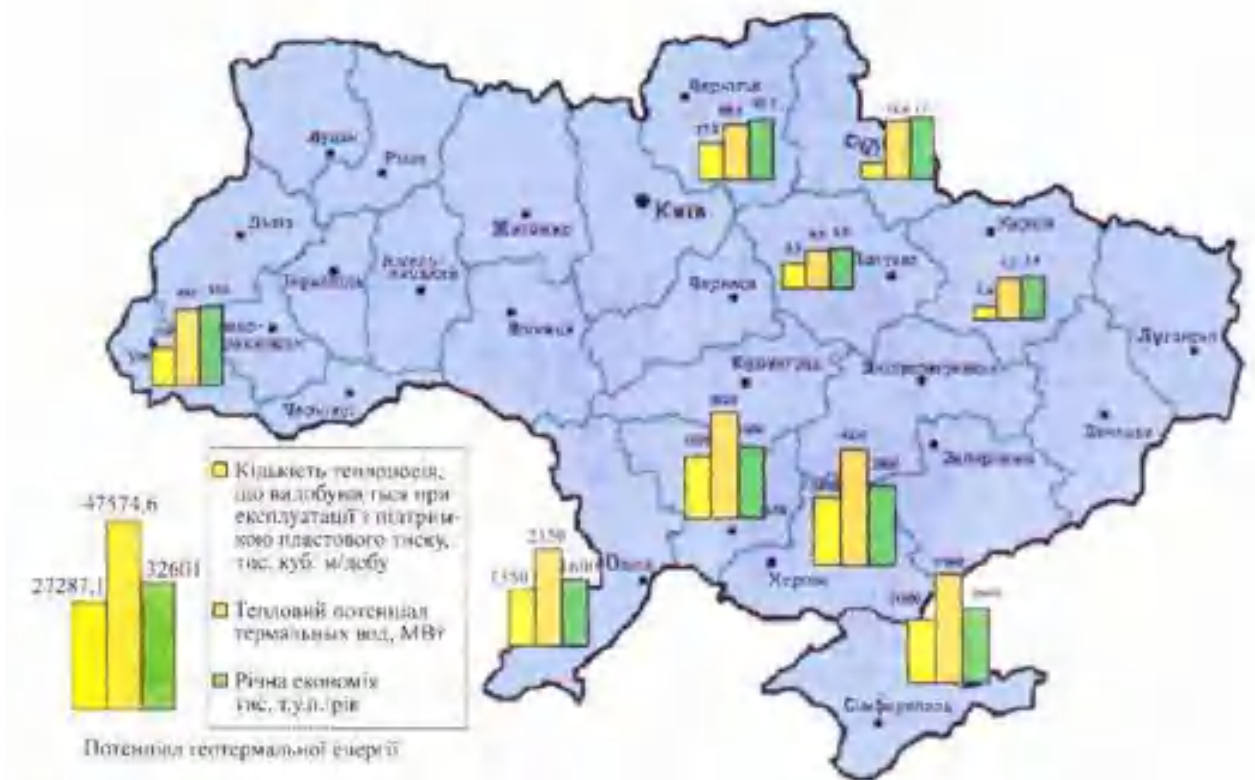
Рис. 5. Загальний потенціал геотермальної енергії України
