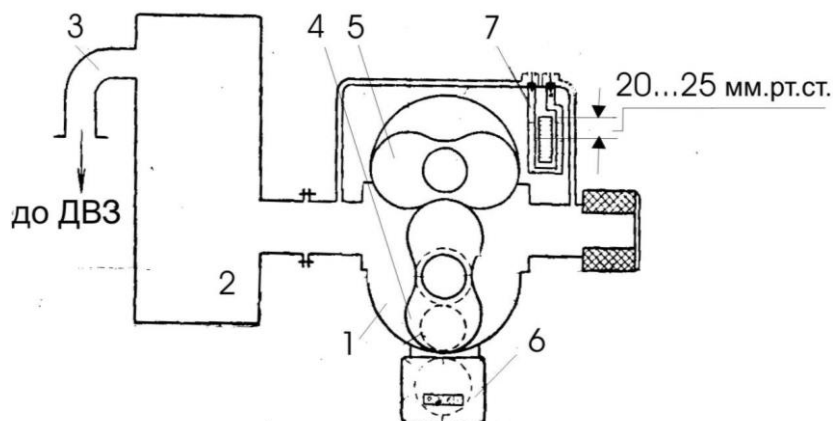
Рис. 5.3 Схема пристрою для вимірювання витрати повітря
