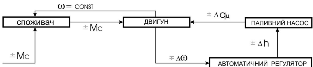
Рис. 1.1. Структурна схема двигуна як об'єкта регулювання
