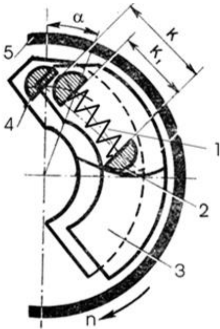
Рис. 1.3. Схема дії автоматичної муфти зміни кута випередження подачі палива:
