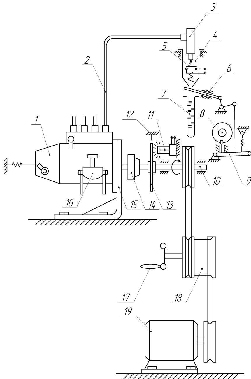
Рис. 2.1. Схема випробувального стенда КИ-921М (СДТА-2)
