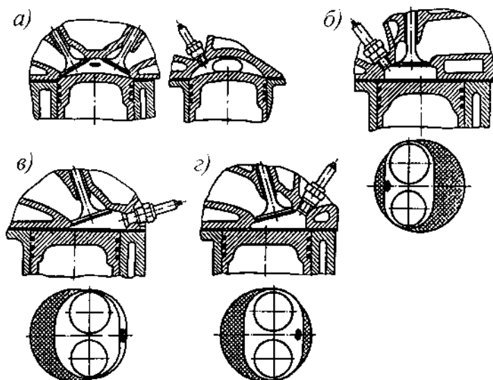
Рис. 2.3 - Схеми деяких типів камер згорання карбюраторних двигунів:
