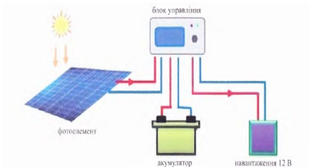
Рис. 1.37. Структурна схема геліоустановки: фотоелемент, акумулятор з навантаженням 12 В [100]
