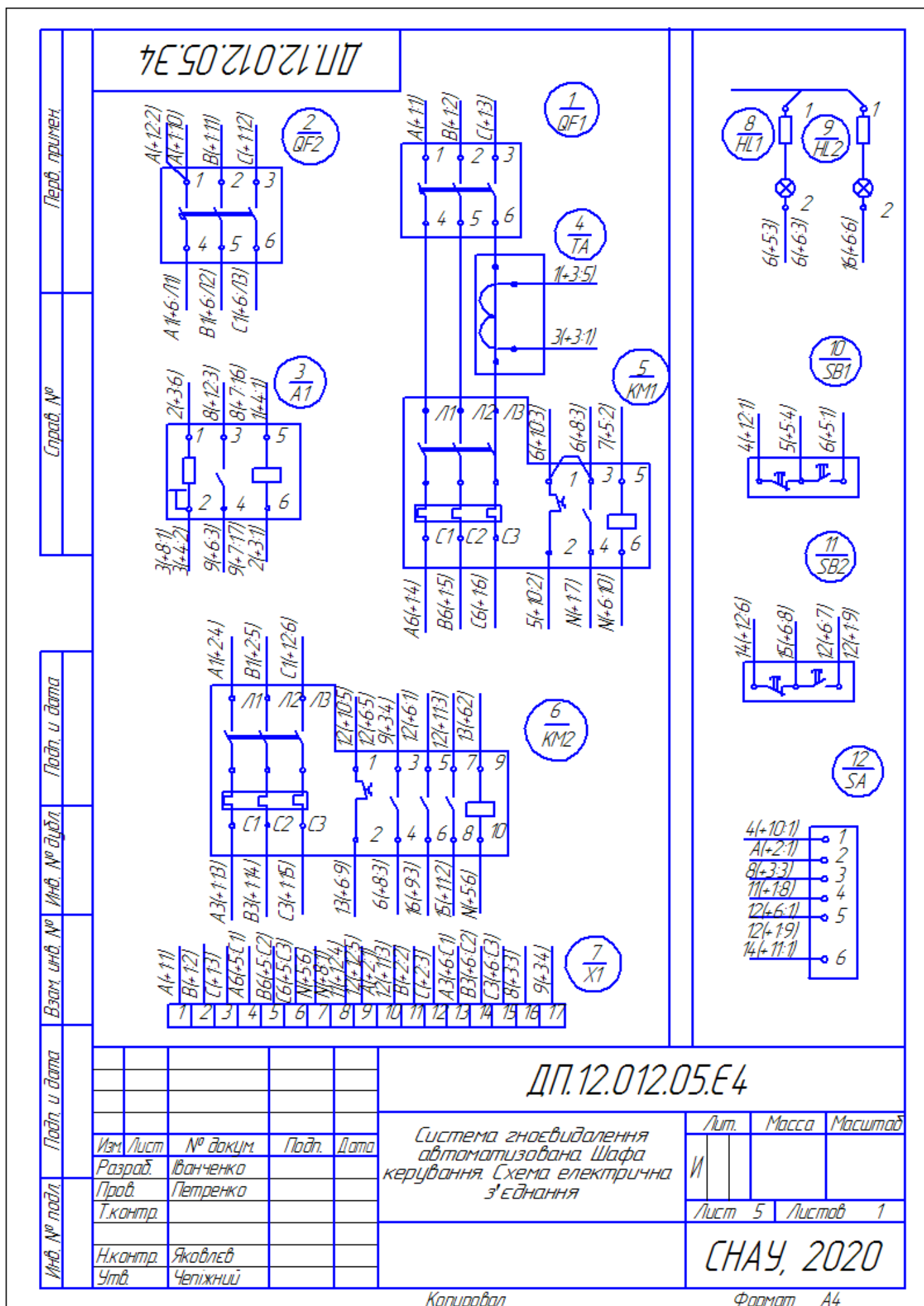
Рисунок В1.5 – Приклад виконання схеми електричної з'єднань автоматизованої системи гноевидалення
