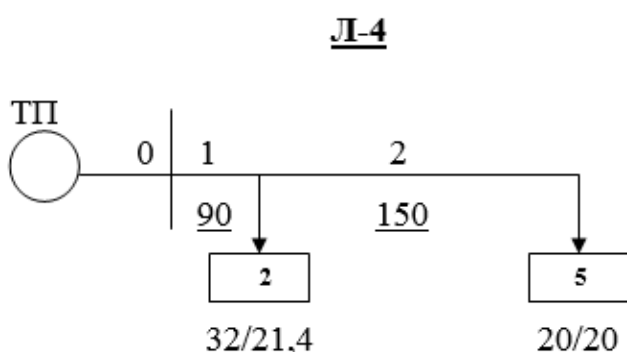
Рисунок Б6.1 – Розрахункові схеми ПЛ-0,38 кВ
