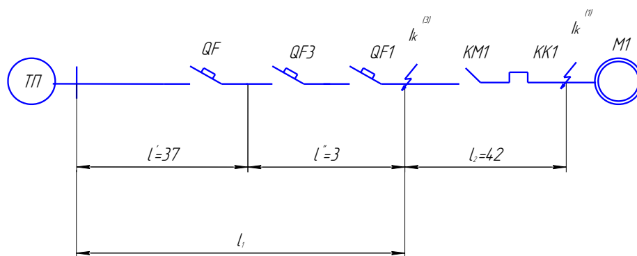
Рисунок Б5.2 – Схема для розрахунку струмів короткого замикання
