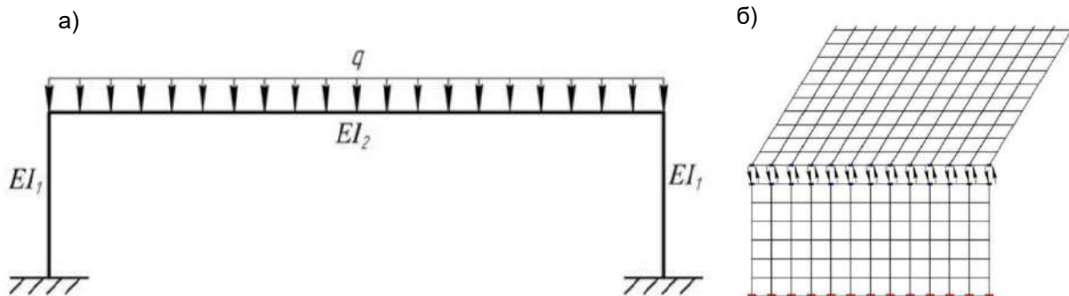
Рис. 1. Загальний вигляд розрахункової схеми –а; об'єднання переміщень суміжних вузлів плити та стіни вузлів–б[2]
